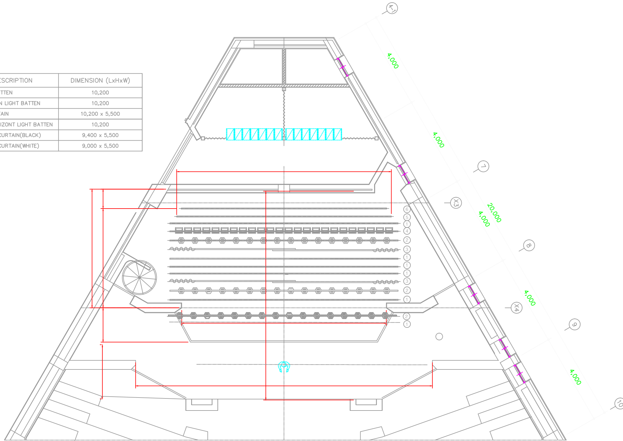
비슬홀 무대 평면도 A3: 1/100 A1: 1/50
